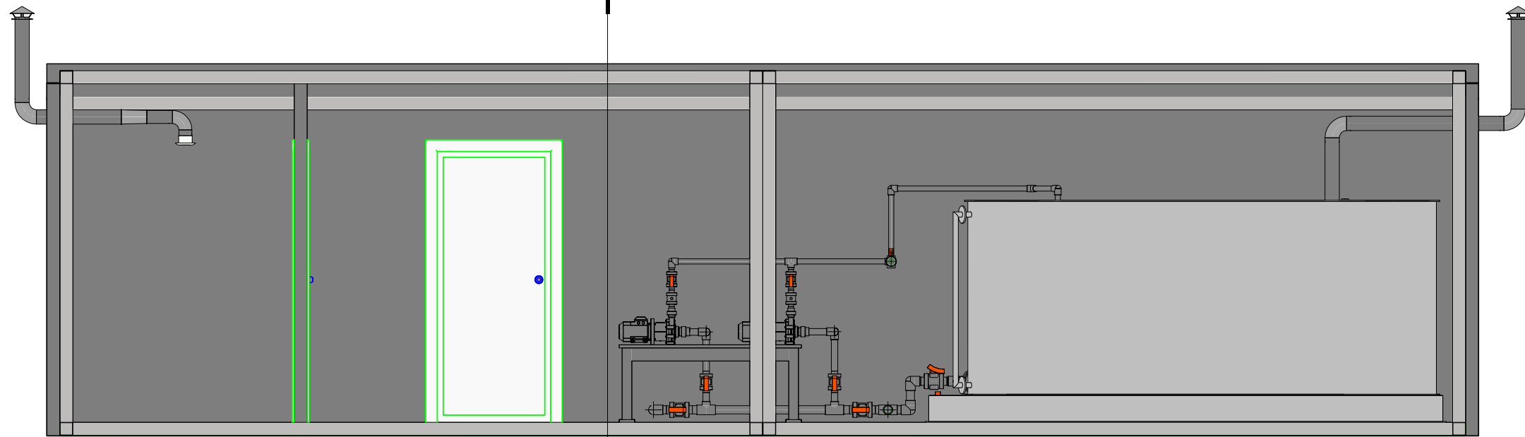
Разрез 3-3
